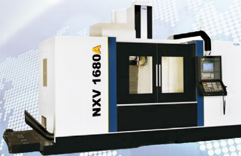
▲ 生產設備>CNC五軸加工機 行程:X軸:1,630mm Y軸:762mm Z軸:700mm 精度:5µm
