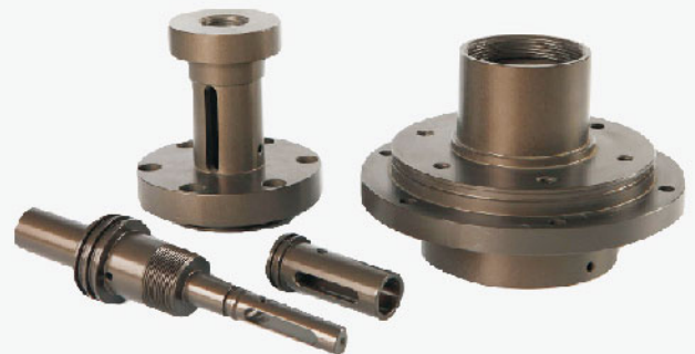
品名：傳動軸套 產品材質：鈦合金 尺寸精度：0.005~0.03mm 產品應用：發動機
